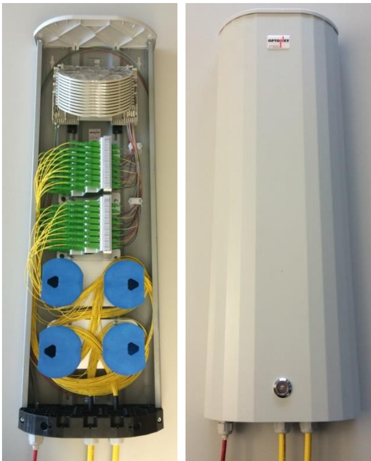
OptoPoint TWO Typ U mit Bodentyp I ▪ 2x Steckerplatte: 24x E2000/APC ▪ 2x Kabelüberlängenmanagement
