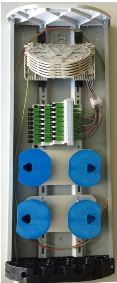
OptoPoint TWO Typ D mit Bodentyp I - 1x Steckerplatte: 24x E2000/APC - 2x Kabelüberlängenmanagement
