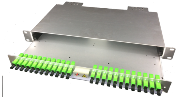
19" 1HE OptoBreak 24x E-2000/APC
